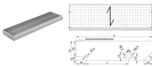
Feuerverzinkte Gitterrost-Treppenstufe, Maschenweite 3 x 3 cm, mit Sicherheits-Antrittskante
